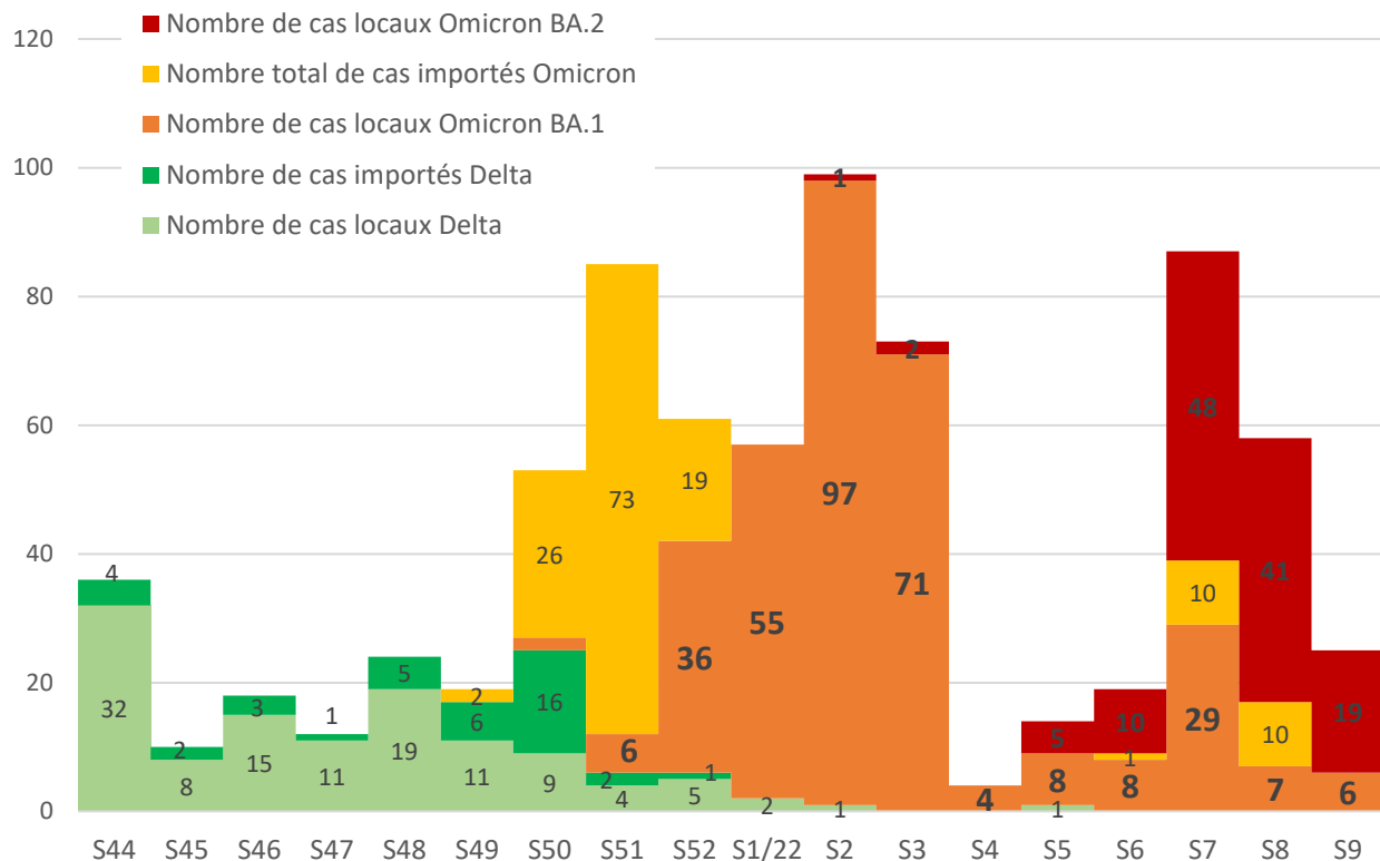
Figure 3. Répartition des types de variants parmi les souches criblées, S44/21 à S9/22
